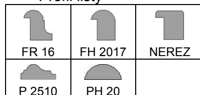
Profil lišty
